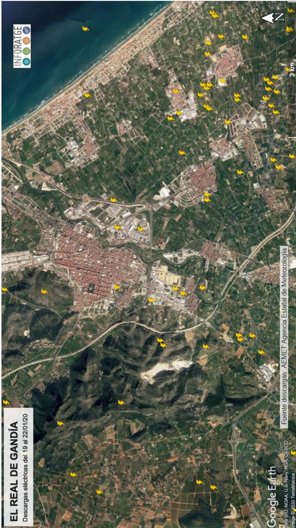
Geolocalización de las descargas eléctricas ~ nube-tierra ~ registradas en el término municipal de EL REAL DE GANDÍA y alrededores entre el 19 y el 22/01/20 Fuente descargas: AEMET Agencia Estatal de Meteorología
