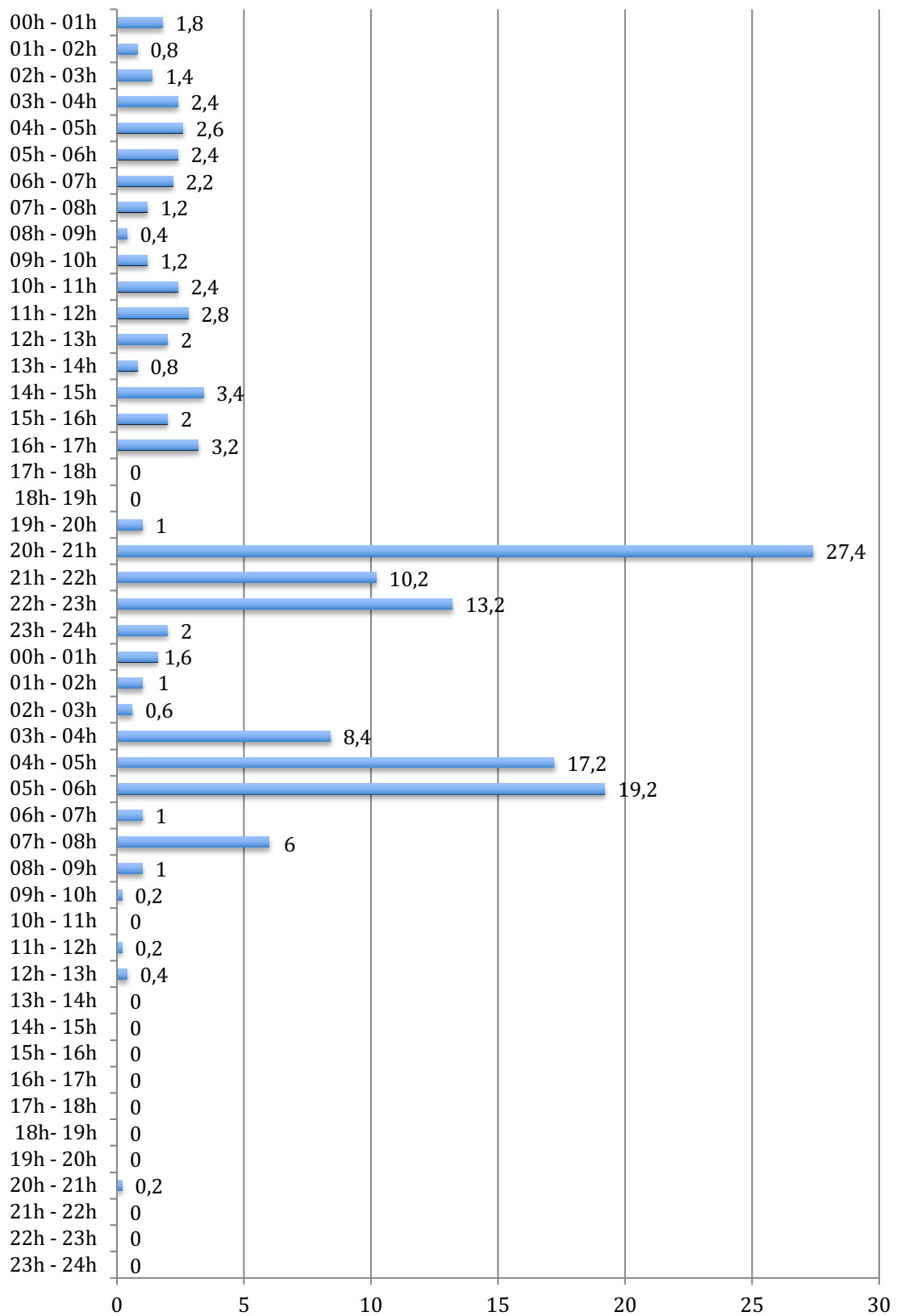
Cantidades de lluvia registradas por horas en EL REAL DE GANDÍA los días 20 y 21/01/20 (en l/m²)
